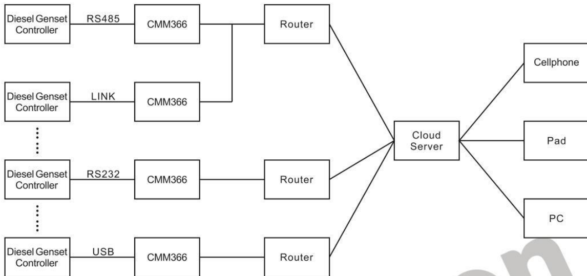
图 1 CMM366-ET System Diagram
